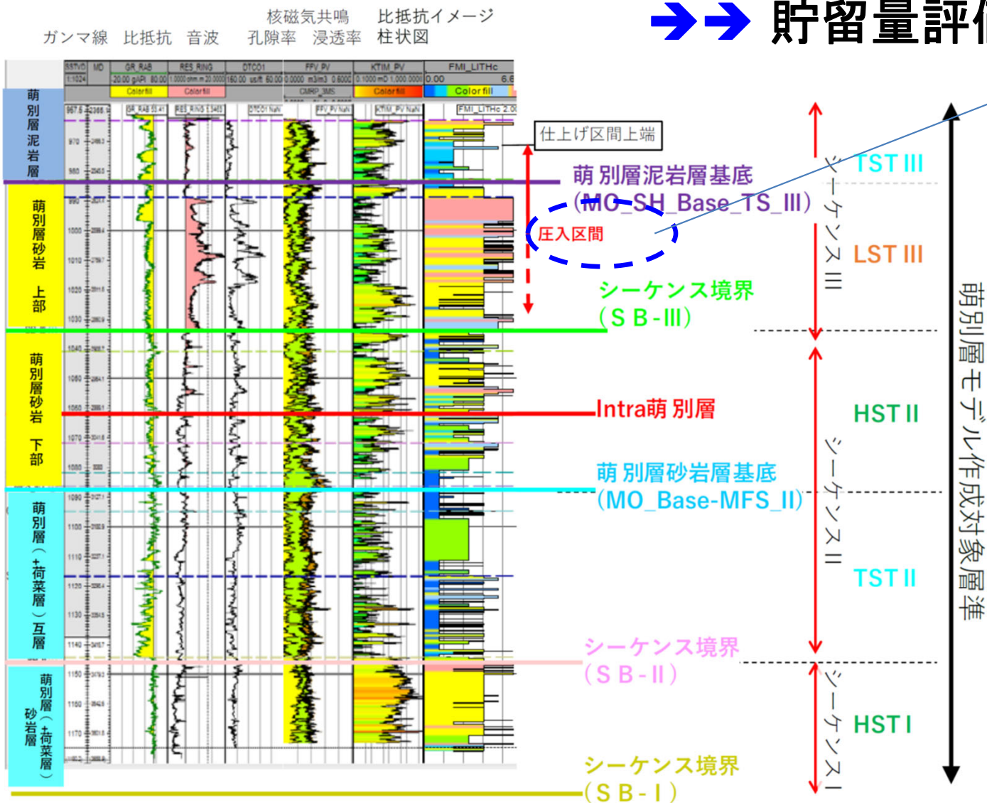
萌別層圧入井 IW-2 における層序区分
